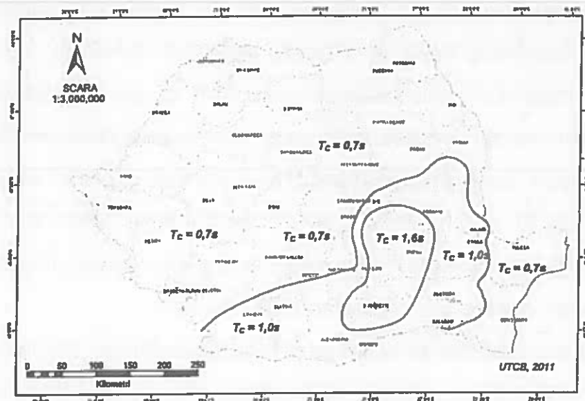
Fig.1 Zonarea teritoriului României în termeni de perioadă de control (colț), T_c a spectrului de răspuns
