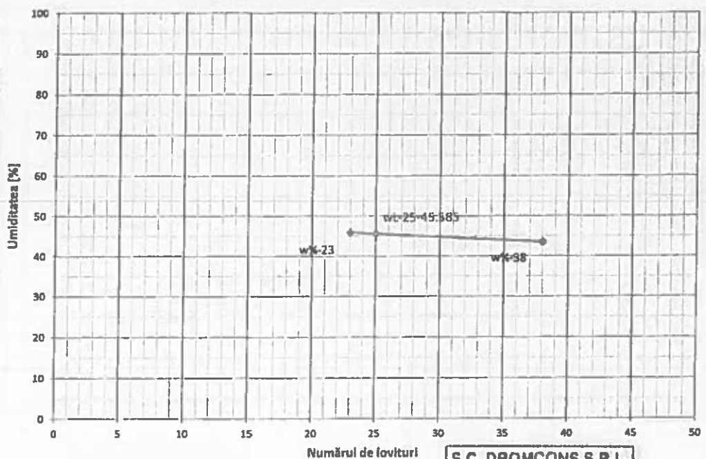
Grafic pentru stabilirea limitelor superioare de plasticitate
